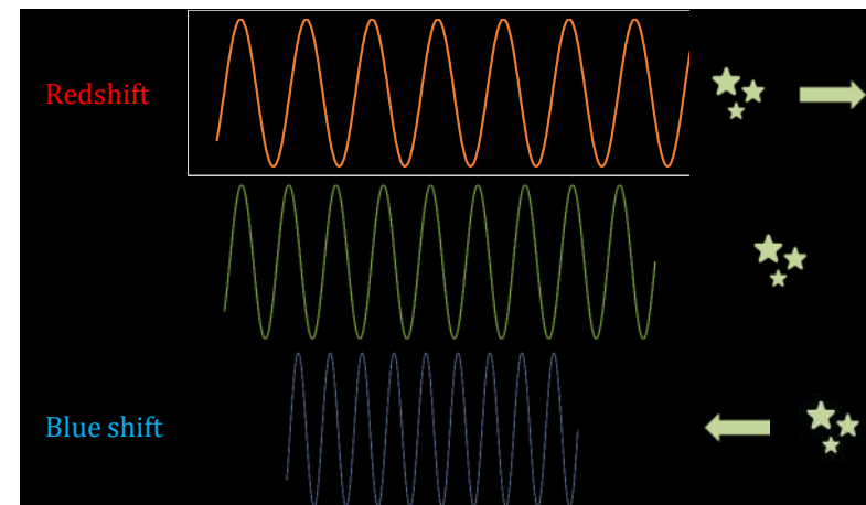
A10.2 - Blue shift and redshift
